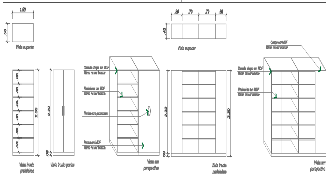
MOBILIÁRIO 5 - Armário grande ESCALA 1/40
