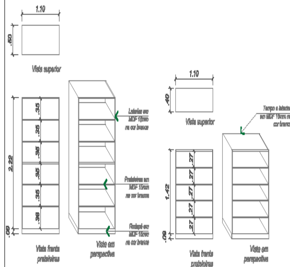
MOBILIÁRIO 6 - Armário prateleira ESCALA 1/40
